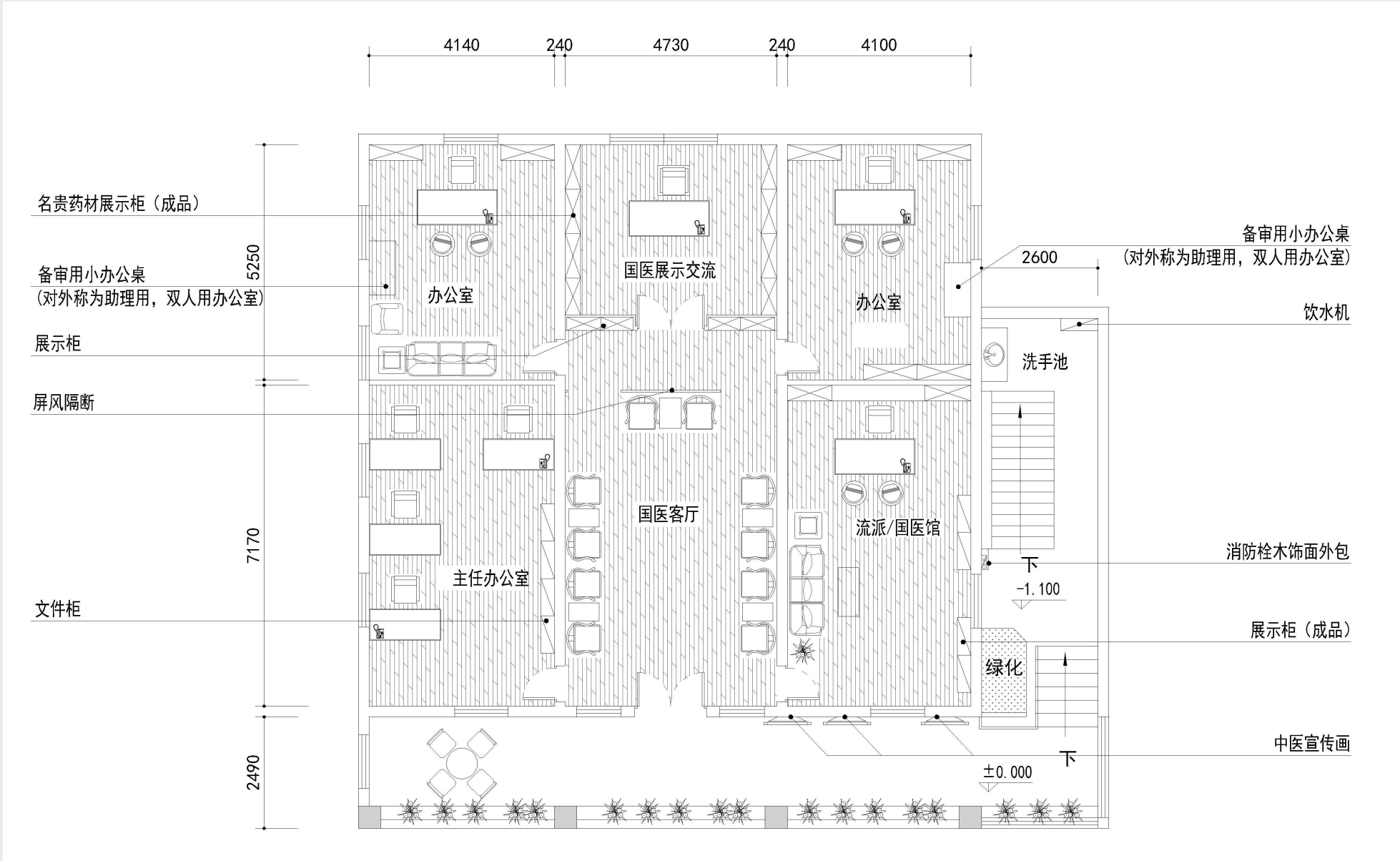
二层平面图
