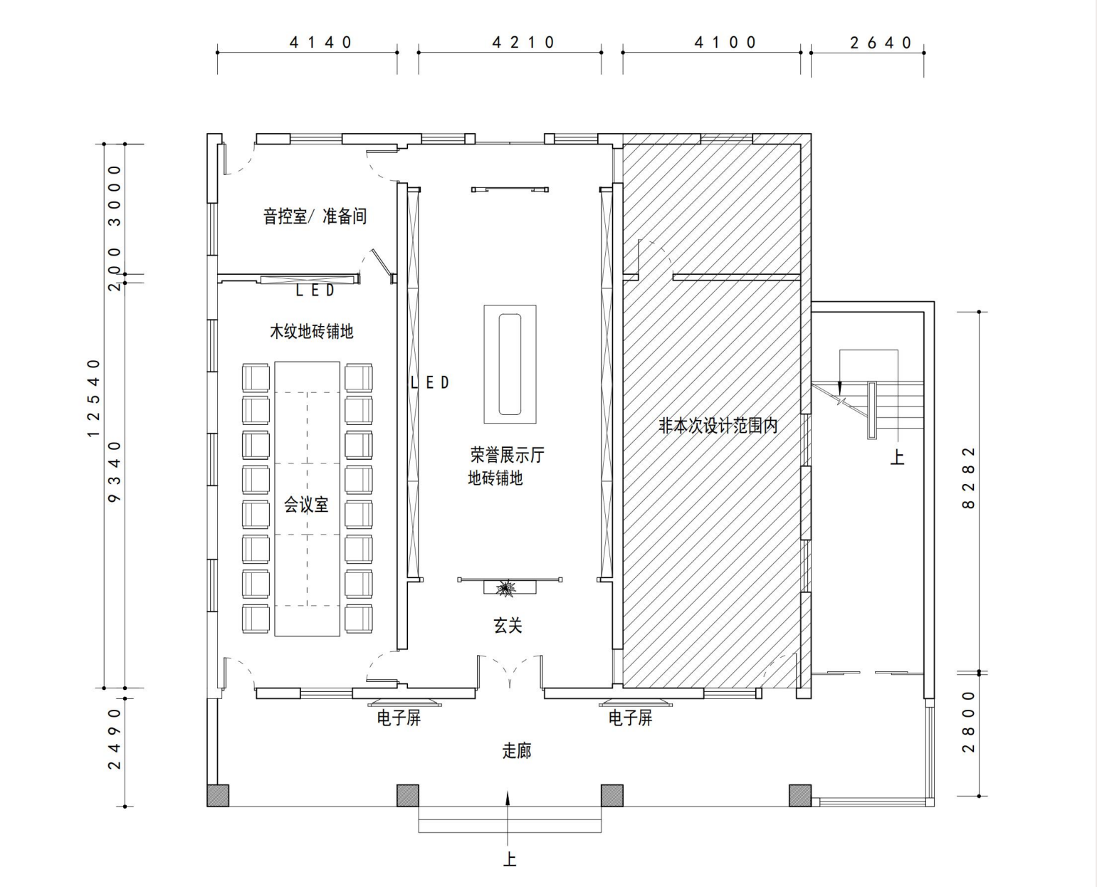
一层平面图
