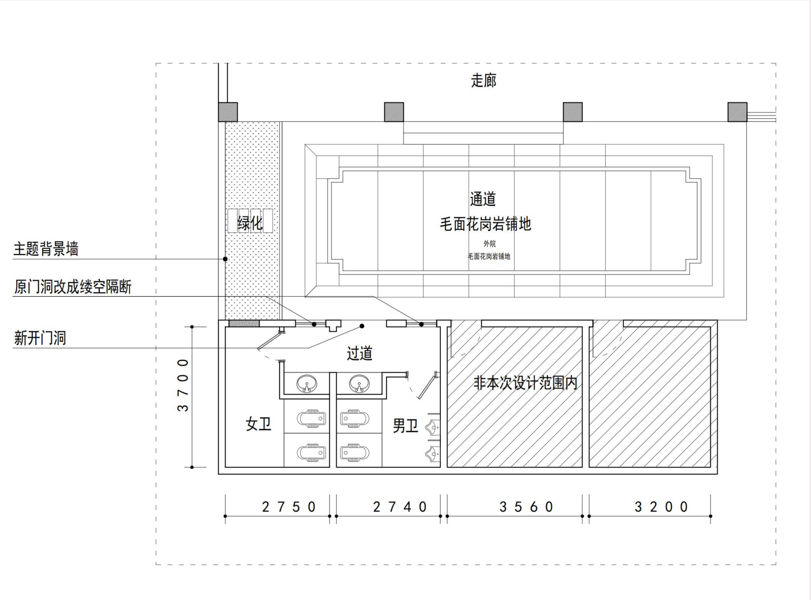
一层卫生间和外庭平面图
